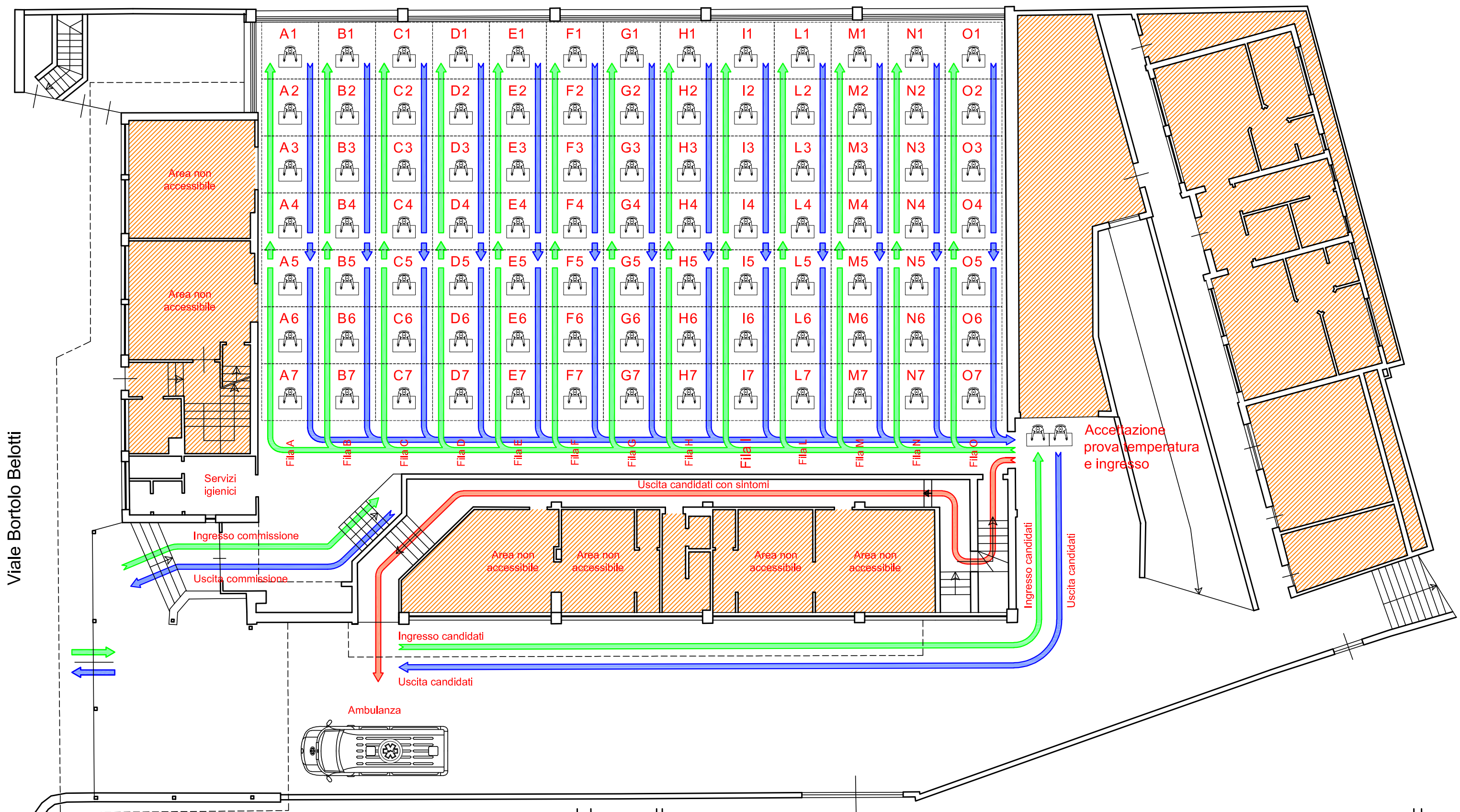
Planimetria sede concorsuale Piano terra e seminterrato
